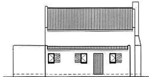
ELEVATION C 1:100
