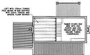
PLAN - LOFT 1:100
